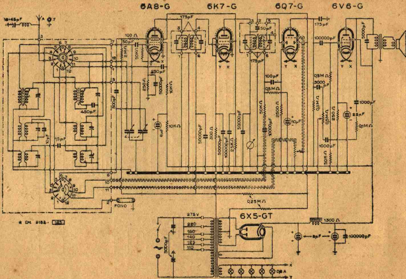
Lo schema elettrico del Siare RR 27
